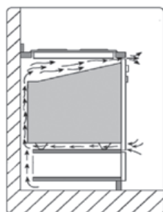
Рис. 7. Схема по встраиванию духового шкафа
