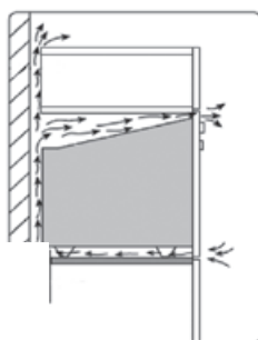
Рис. 7. Схема по встраиванию духового шкафа
