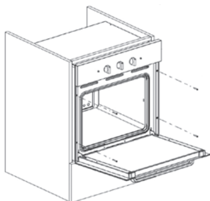
Рис. 7. Схема по встраиванию духового шкафа
